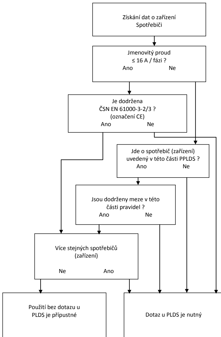
Obr. 1 Schéma po posuzování přístrojů/zařízení se zřetelem na elektromagnetickou kompatibilitu (EMC)
